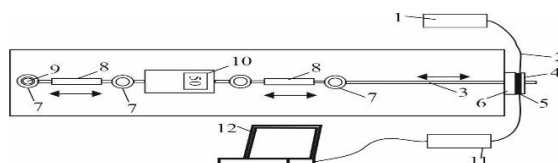
1 - источник света, 2 - чувствительный элемент, 3 – натяжная шпилька, 4 – подвижный диск, 5 – демпфер, 6 – неподвижный диск, 7 - соединительное кольцо, 8 - натяжная муфта, 9 - неподвижная опора, 10 - измеритель нагрузки, 11 – телевизионная матрица, 12 - компьютер
