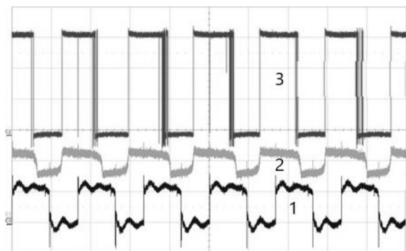
Рис.2 Осциллограммы приемного модуля для УФ-связи на основе \text{Ga}_2\text{O}_3 . 1 – импульсы на светоизлучающем диоде; 2 – сигнал на выходе усилителя; 3 – сигнал на выходе компаратора. Масштаб – 10 мкс на клетку.
