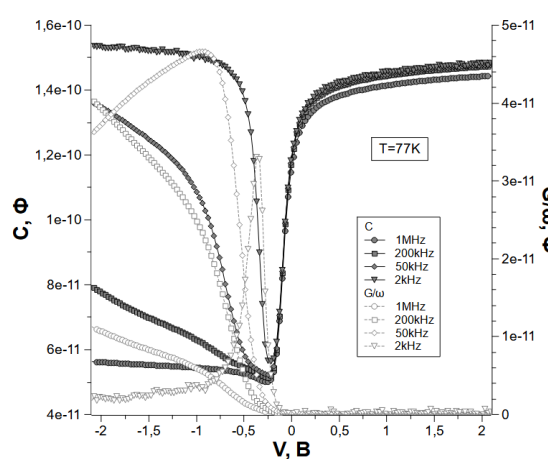
Рисунок 4 — ВФХ и зависимости от напряжения смещения нормированной на циклическую частоту дифференциальной проводимости структуры № 2, измеренная при прямой развертке напряжения при температуре 77 К. Прямая развертка
