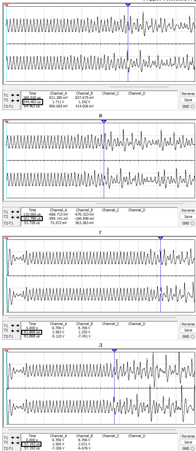
рис.2. Осциллограммы колебаний при разрушении синфазного режима R_3=0.05 Ом: а) R_{CB}=16.3 Ом; б) R_{CB}=11.2 Ом; в) R_{CB}=10.2 Ом; г) R_{CB}=9.1 Ом; д) R_{CB}=5 Ом; е) R_{CB}=2 Ом
