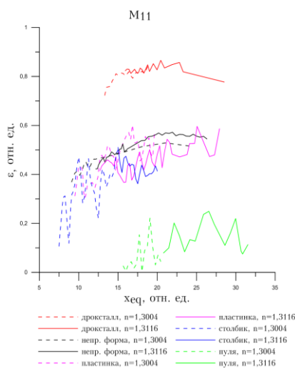
рис. 1. Относительная ошибка дифференциального сечения рассеяния ( M_{11} ) в зависимости от параметра размера частиц в направлении рассеяния назад на показателях преломления 1.3116 и 1.3004 (пунктир)
