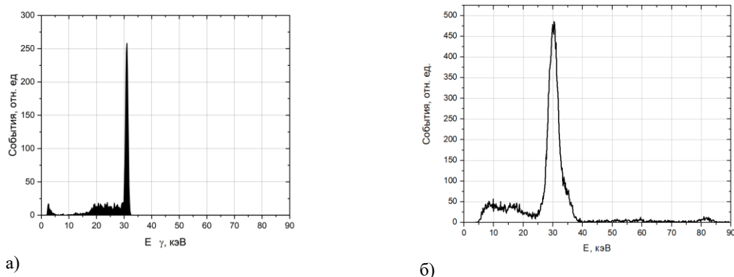
рис. 1 Сравнение экспериментального и расчетного амплитудного спектра для 31 кэВ: а) расчетный амплитудный спектр; б) экспериментальный амплитудный спектр ^{133}\text{Ba}
